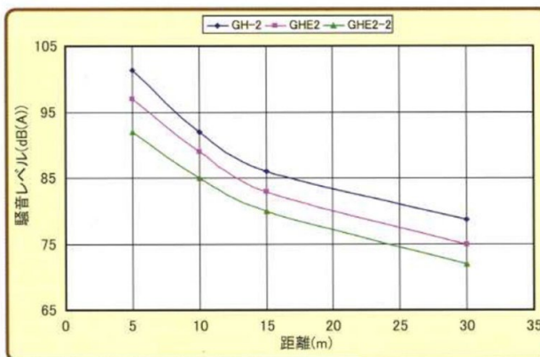
● GHE2-2 騒音レベル(dB(A))
